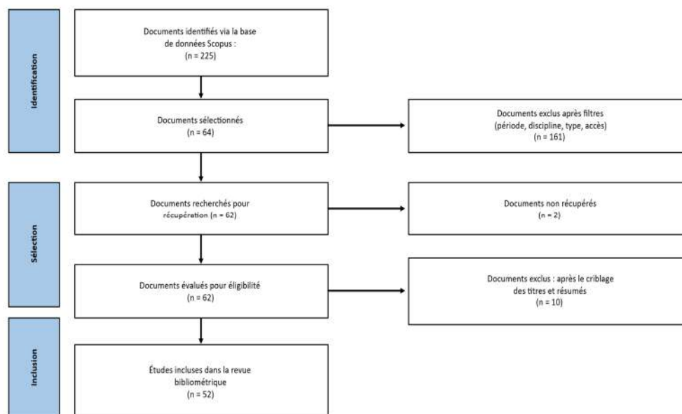
Figure 1 : Diagramme de flux PRISMA indiquant le déroulement de la recherche dans l'identification et le filtrage des sources pour l'analyse bibliométrique
